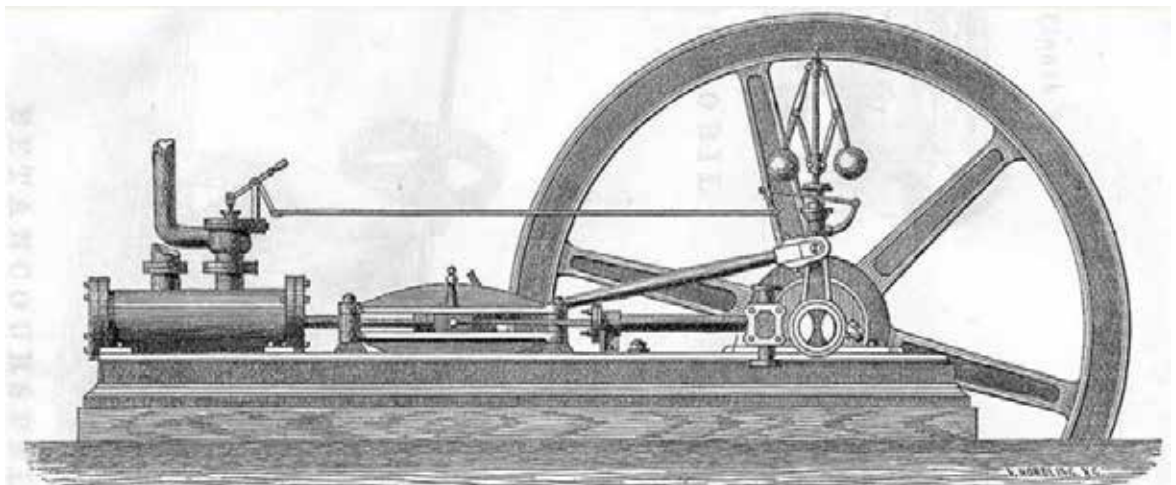
FÖRBÄTTRAD HORISONTEL ÅNGMACHIN
